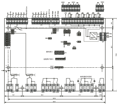
标准接线图
