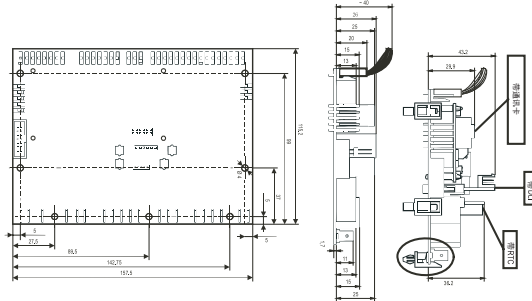
尺寸 (mm)
